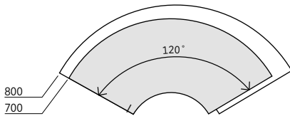
120° with intercut | 120° Beidseitig gerundet
