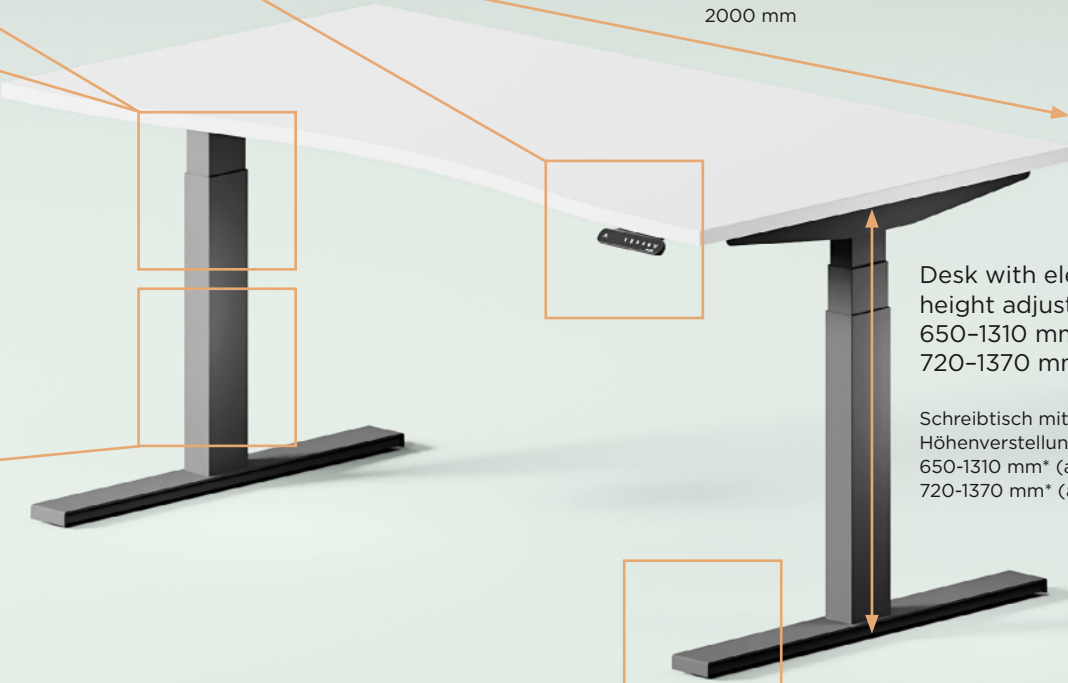
Total width up to 2000 mm Gesamtbreite bis 2000 mm
