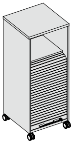
1263 × 480 × 480 mm
