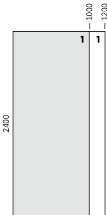
3. Bench for high table, O-leg | Sitzbank für Hochtisch mit Kufengestell
